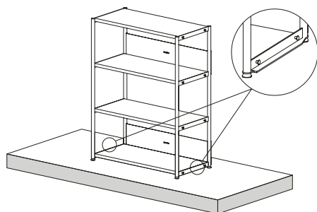
UNIT ground mount Accroche au sol UNIT
